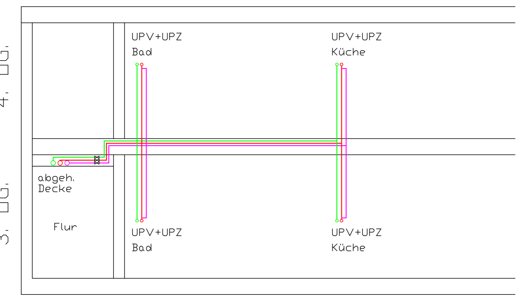
Systemdarstellung Wasserverteilung
